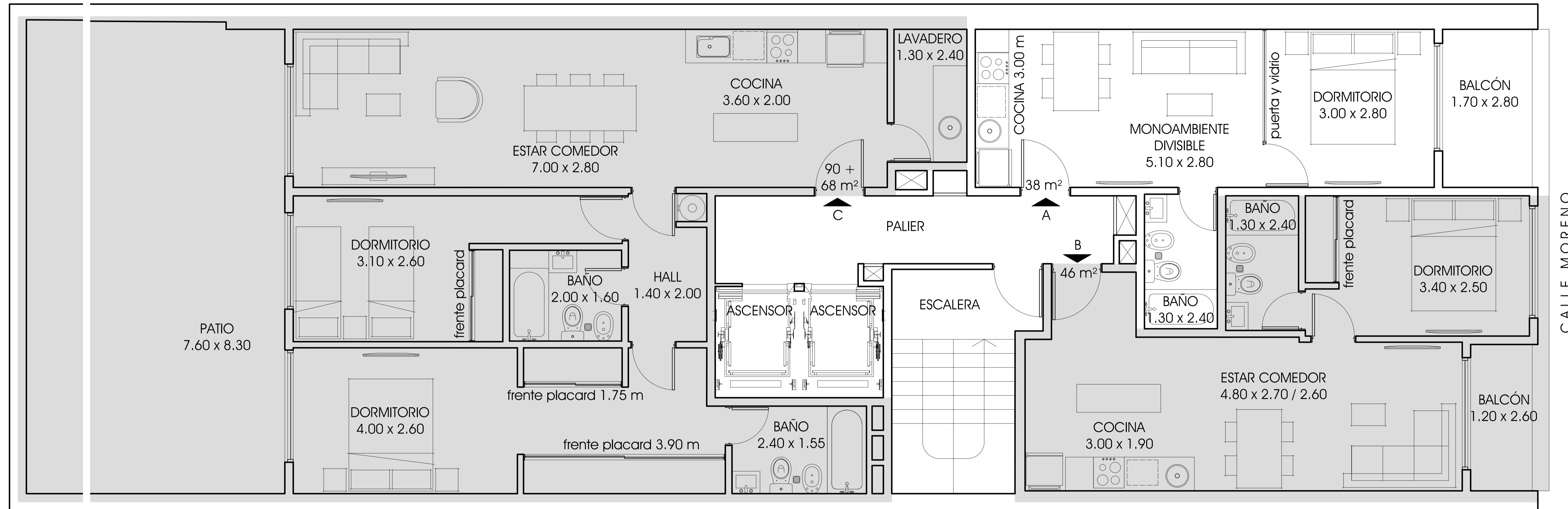
PLANTA 1º PISO
